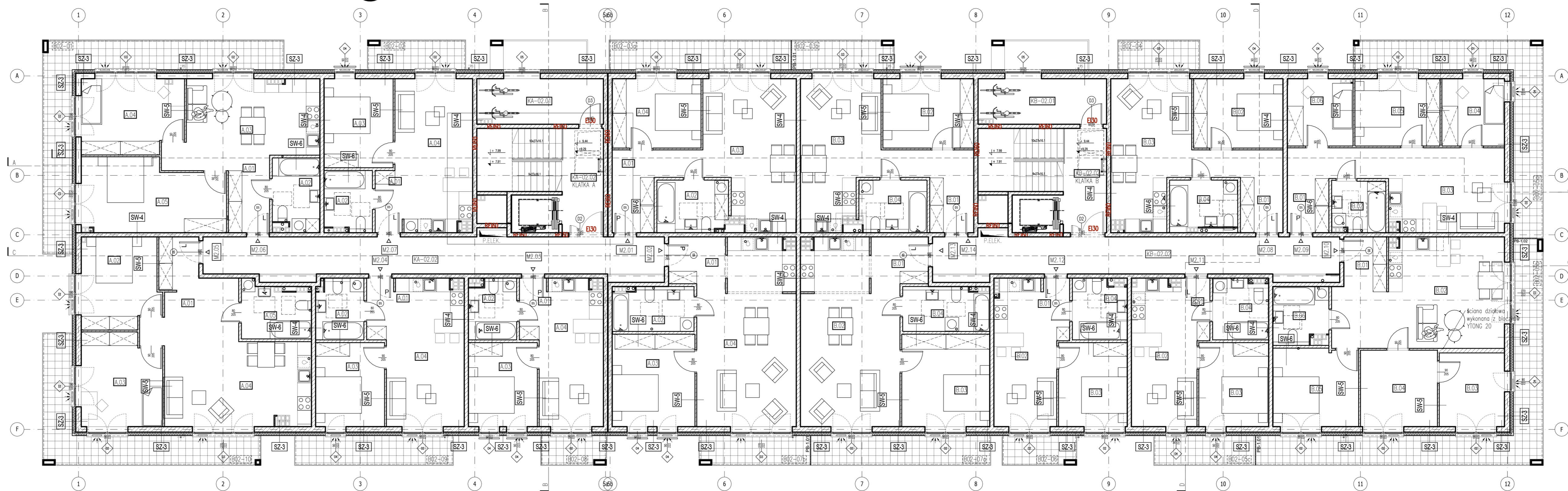
RZUT KONDYGNACJI NR 4 SKALA 1:100
